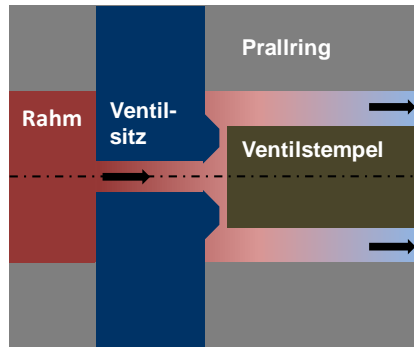
konv. Flachventil
